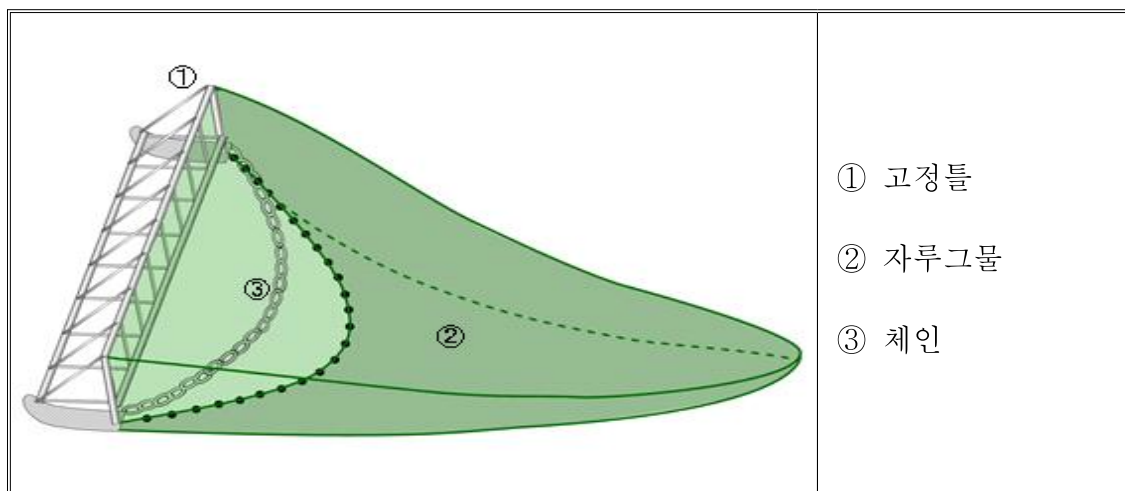
근해형망 어구 겨냥도
