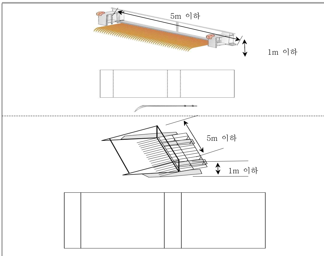
패류형망 표준어구 구성도
