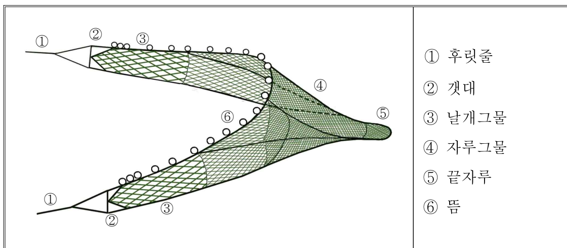
동해구외끝이중형저인망 어구 겨냥도
