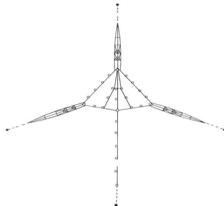
- 삼각망 -
