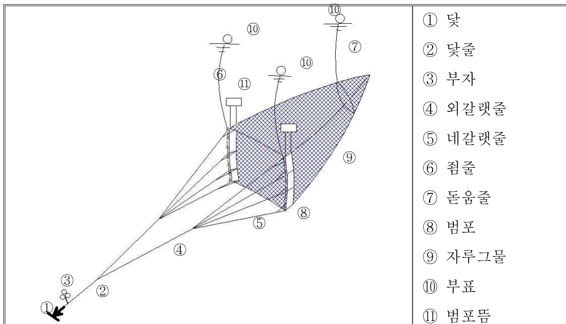
연안개량안강망 어구 겨냥도
