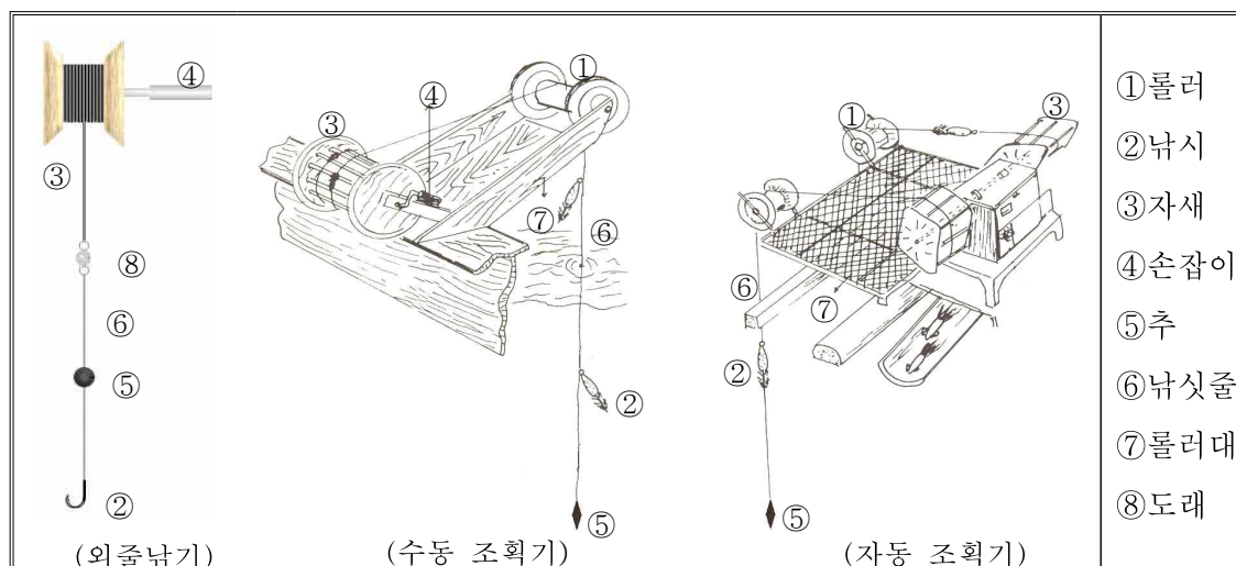
근해채낚기 어구 겨냥도
