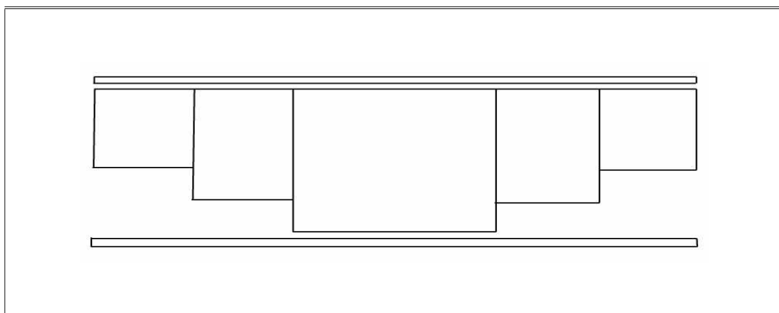
연안선망 표준어구 구성도
