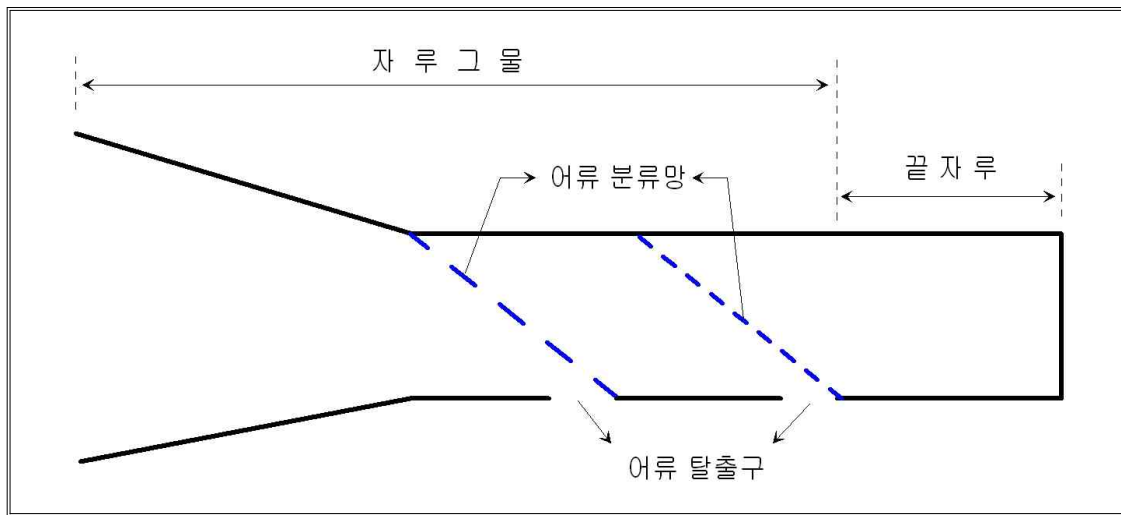
근해안강망 어류분류망 구성도
