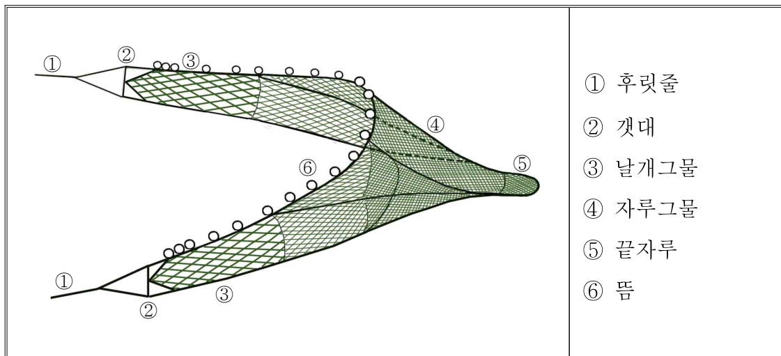
서남해구의끝이중형저인망 어구 겨냥도
