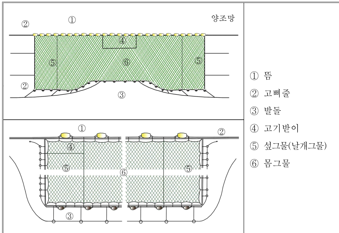
연안선망 어구 겨냥도
