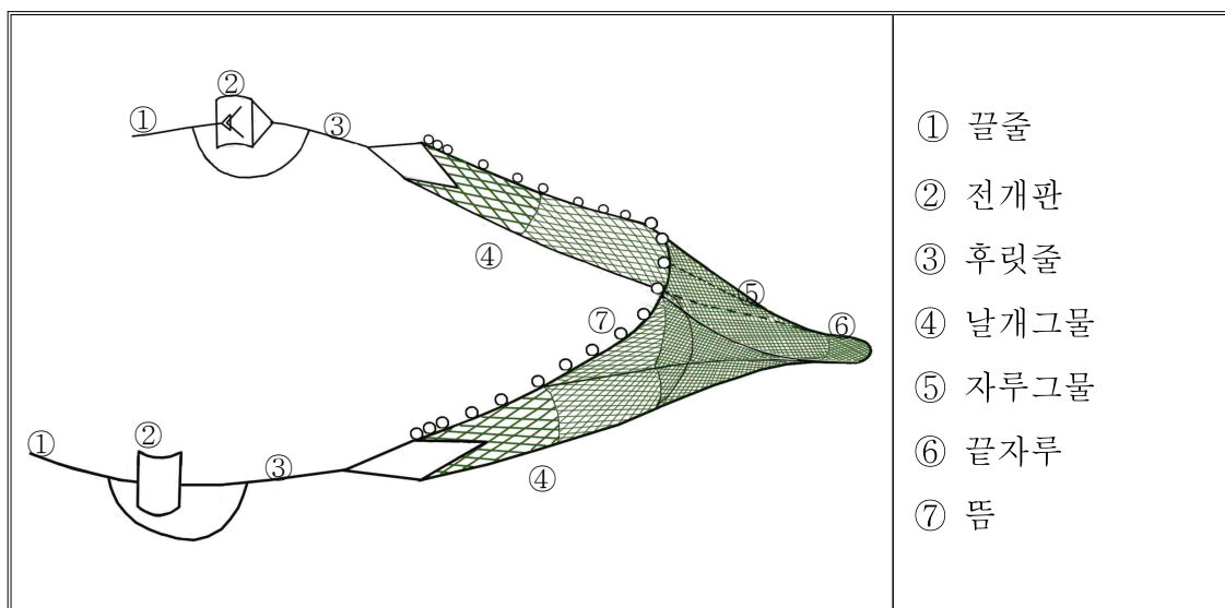
동해구중형트롤망 어구 겨냥도
