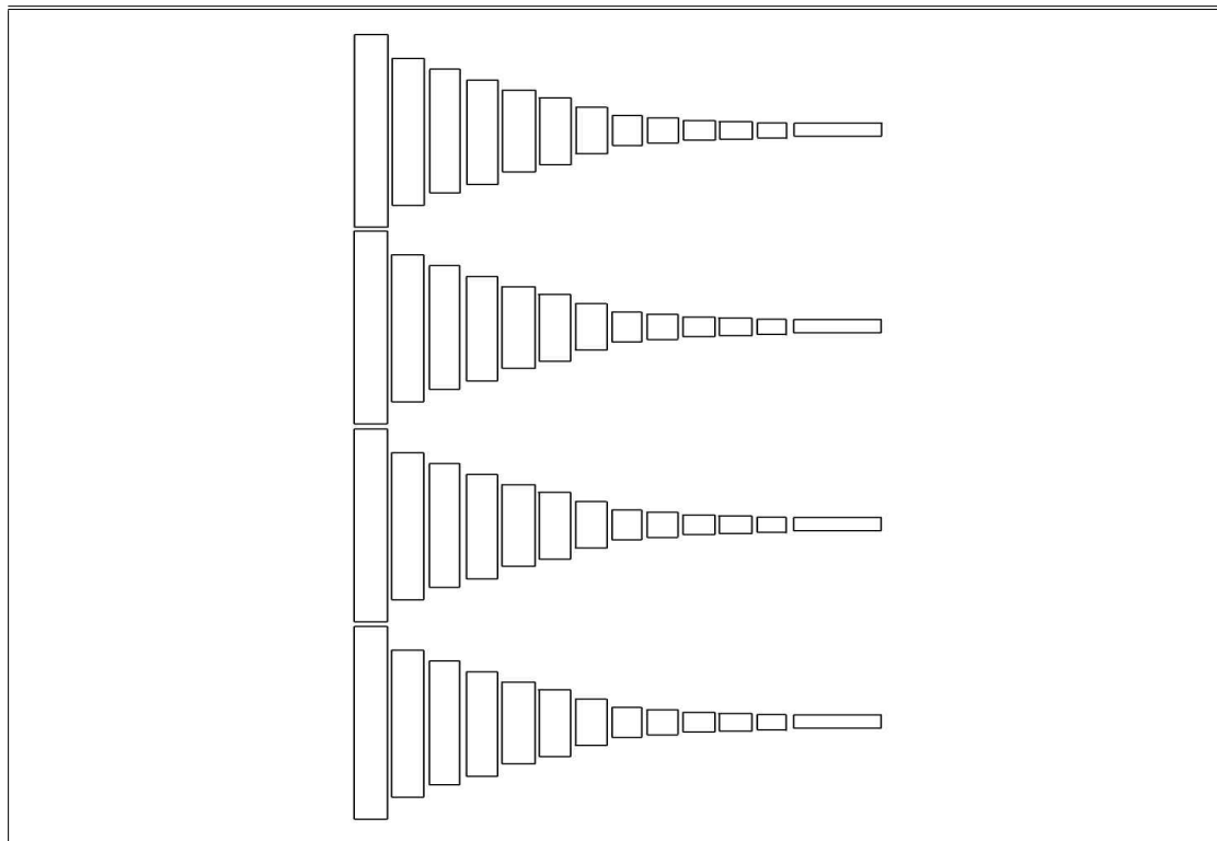
안강망 표준어구 구성도
