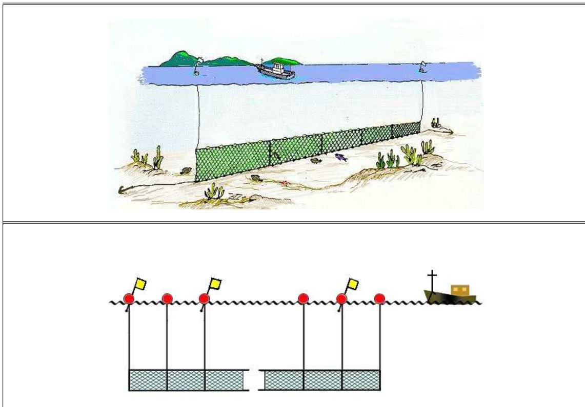
근해자망 조업모식도
