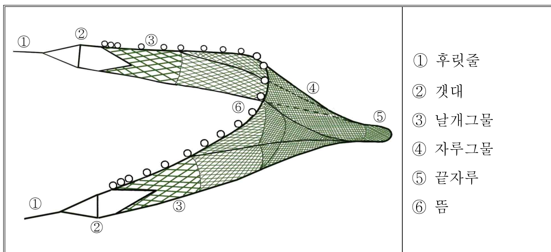
서남해구쌍끌이중형저인망 어구 겨냥도
